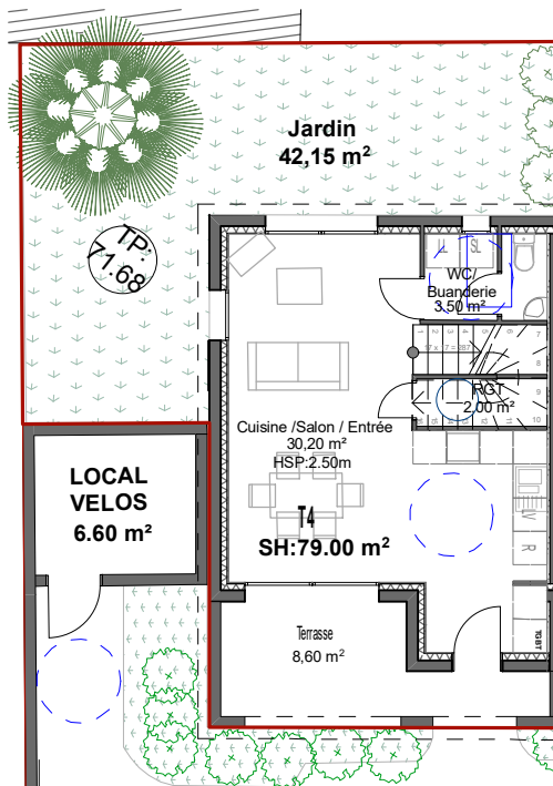
VILLA 1 / RDC Ech: 1/150
